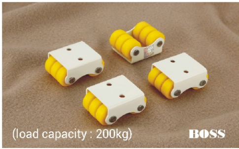
6 WHEEL MOVING CASTER A-117 (PU)
